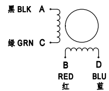
接线图 Wiring Diagram
